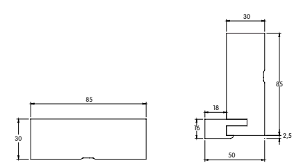
traverse haute ( et basse si option) montant + cache-jeu
